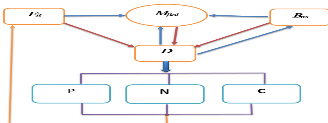
Расми 2. Диаграммаи селии амсилаи концептуалии популятсияи моҳиҳои экосистемаи обанбори “Норак”
